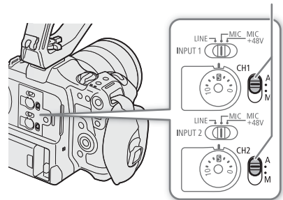
CH1/CH2 音频电平开关
